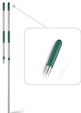
589600 MANICO TELESCOPICO IN ALLUMINIO CON FORO Da cm 102 a 184. Ø esterno cm 2,6 interno cm 2,3
